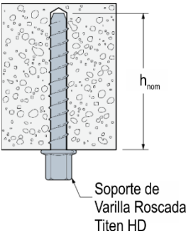
FIGURA 2B— INSTALACIÓN DEL SOPORTE DE VARILLA ROSCADA TITEN HD®
