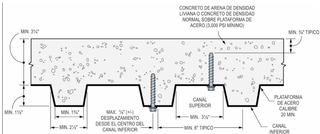
FIGURA 4—INSTALACIÓN DE ANCLAJES DE TORNILLOS DE \frac{1}{4} DE PULGADA DE DIÁMETRO DEL MANGO Y SOPORTES DE VARILLAS ROSCADAS EN EL SOFITO SOBRE PLATAFORMAS DE ACERO PERFILADAS EN ENSAMBLAJES DE PISOS Y TECHOS (1 in = 25.4 mm)
