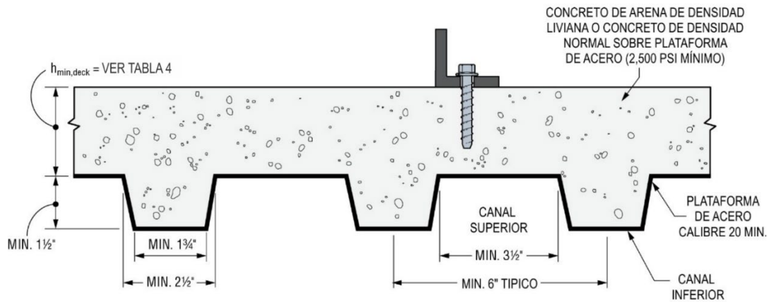
FIGURA 5—INSTALACIÓN DE ANCLAJES DE TORNILLOS DE 1/4 DE PULGADA, 3/8 DE PULGADA Y 1/2 PULGADA DE DIÁMETRO DEL MANGO EN LA PARTE SUPERIOR DE ENSAMBLAJES DE PISOS Y TECHOS DE PLATAFORMAS DE ACERO PERFILADAS RELLENAS DE CONCRETO (1 pulg = 25.4 mm)
